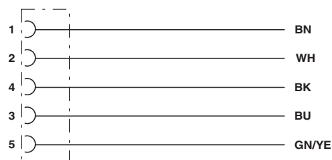
电路图
