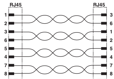
电路图
