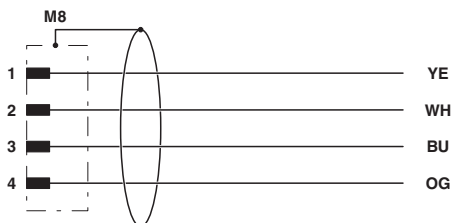
电路图
