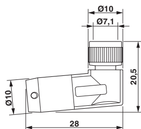
尺寸图
