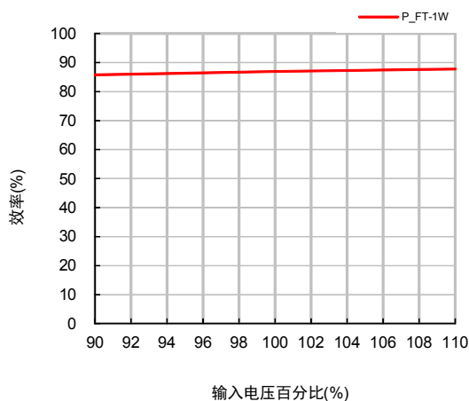
效率与输入电压关系曲线图 (满载)
