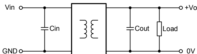
图 1 应用电路图
