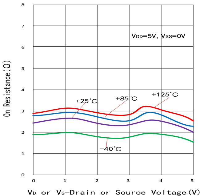
图 3. 单电源不同温度下的 R 和 V_D(V_S) 的关系图
