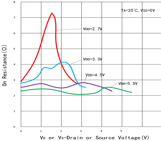
图 1. 单电源下的 R 和 V_D(V_S) 的关系图
