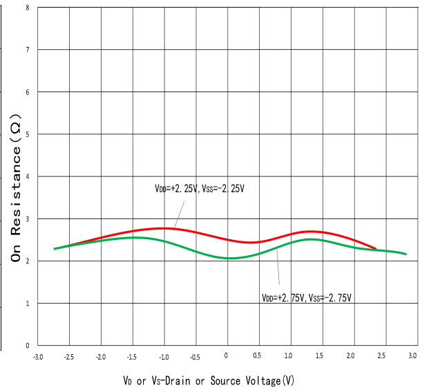
图 2. 双电源下的 R 和 V_D(V_S) 的关系图
