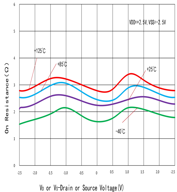
图 4. 双电源不同温度下的 R 和 V_D(V_S) 的关系图
