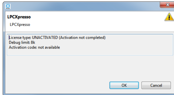
Fig 18. LPCXpresso IDE
