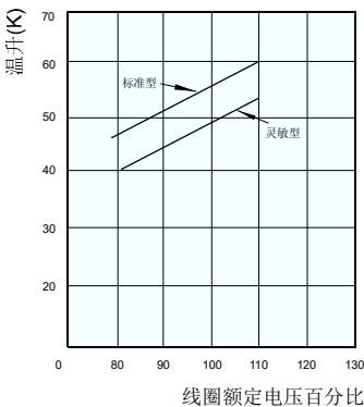
线圈温升
