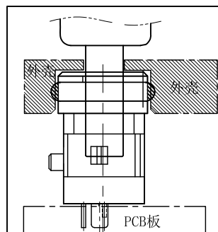
组装示意图
