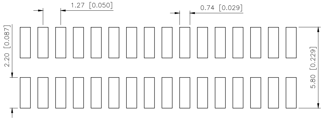
P.C.B LAYOUT
