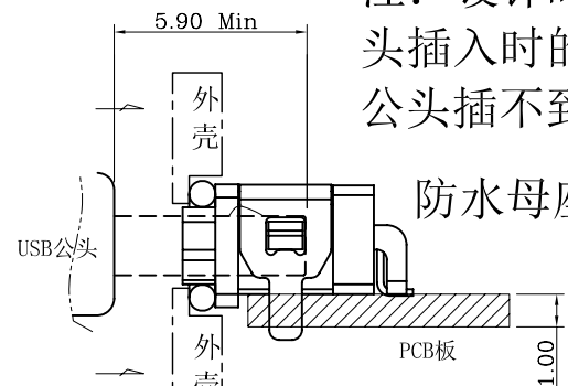
组装示意图
