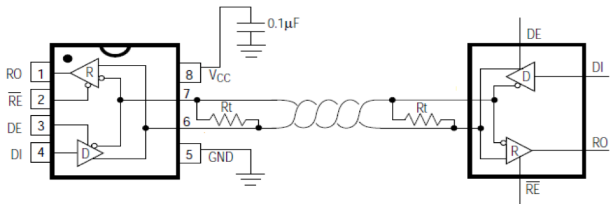
图 1：MAX3483ESA-TD典型半双工应用电路
