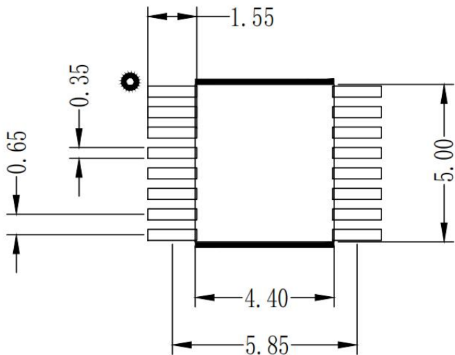
图 3 HWD90LV048A 推荐焊盘图
