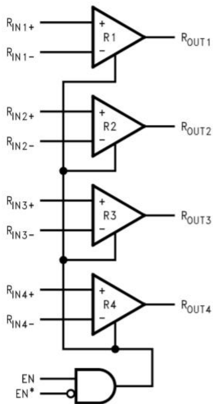
图 1 功能框图
