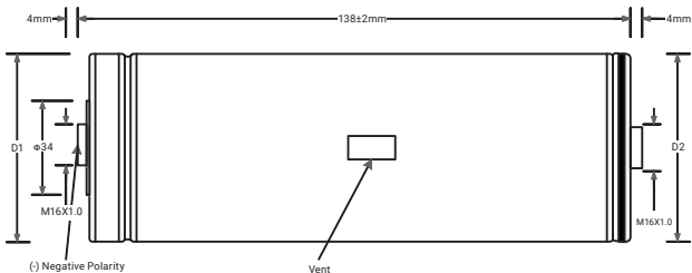
Cylindrical Lug Type 3000F Part
