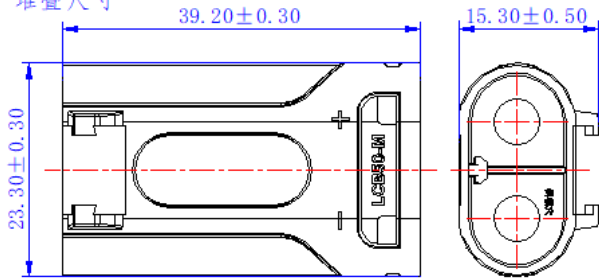
堆叠尺寸
