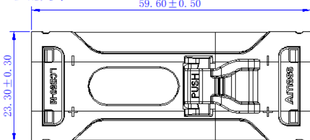
互配尺寸
