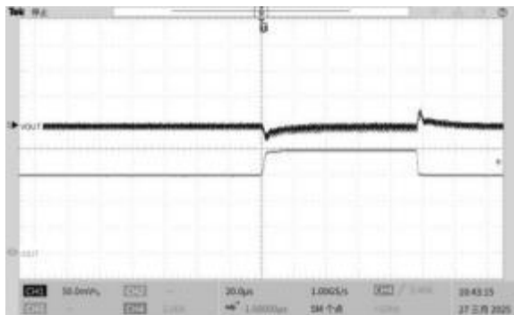
图 6 1.2V 输出瞬态响应
