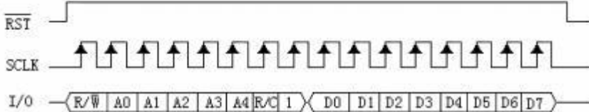
图 3 DS1302ZN数据传送图示
