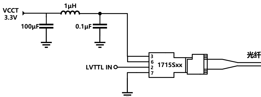
图 4 NRS1715Sxx 典型应用电路图
