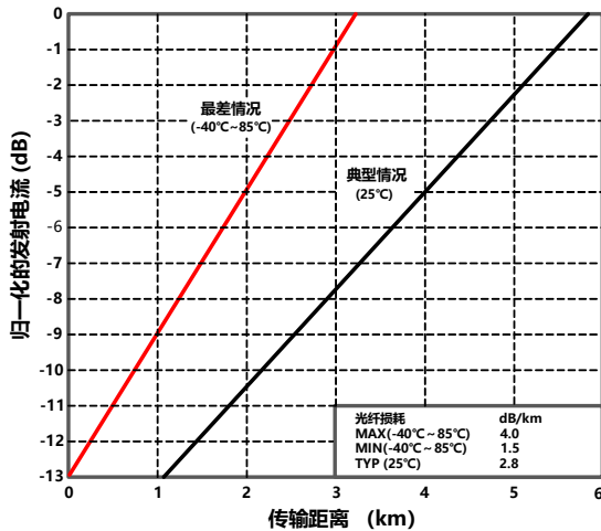
图 5 NRS1715Sxx/2418xx 配合 62.5/125μm 芯径光纤的传输距离极限
