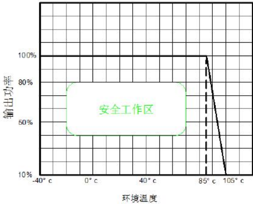
温度曲线图
