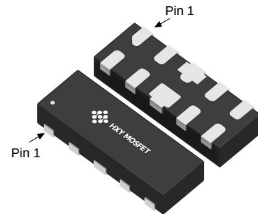
DFN2510-10L (UDFN-10(1x2.5))
