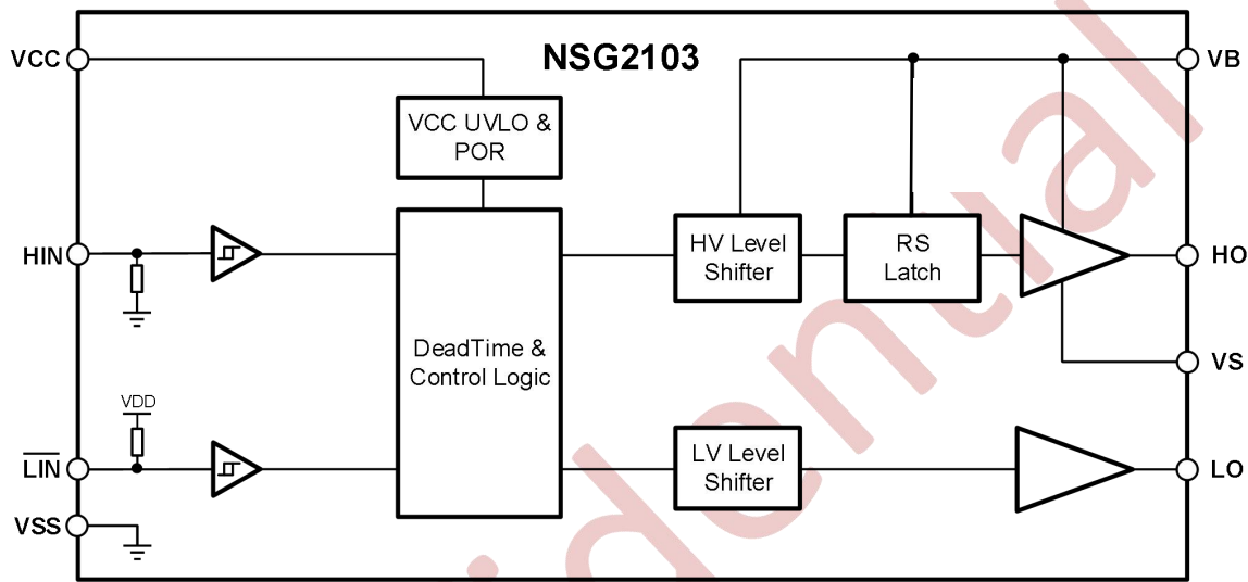
图 10-1 NSG2103 的功能框图
