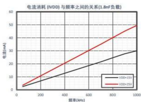
图 4 电流消耗 (IVDD) 与频率间的关系 (1.8nF 负载)
