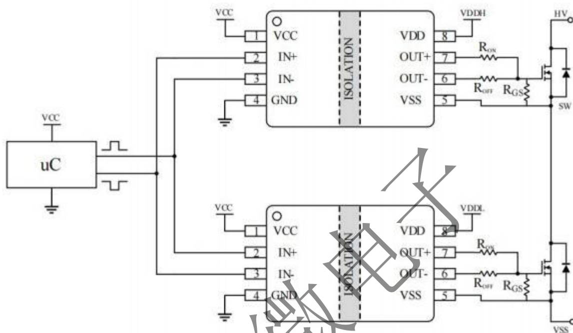
图 29 Interlock 功能
