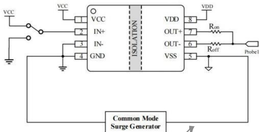
图 26 CMTI 测试电路
