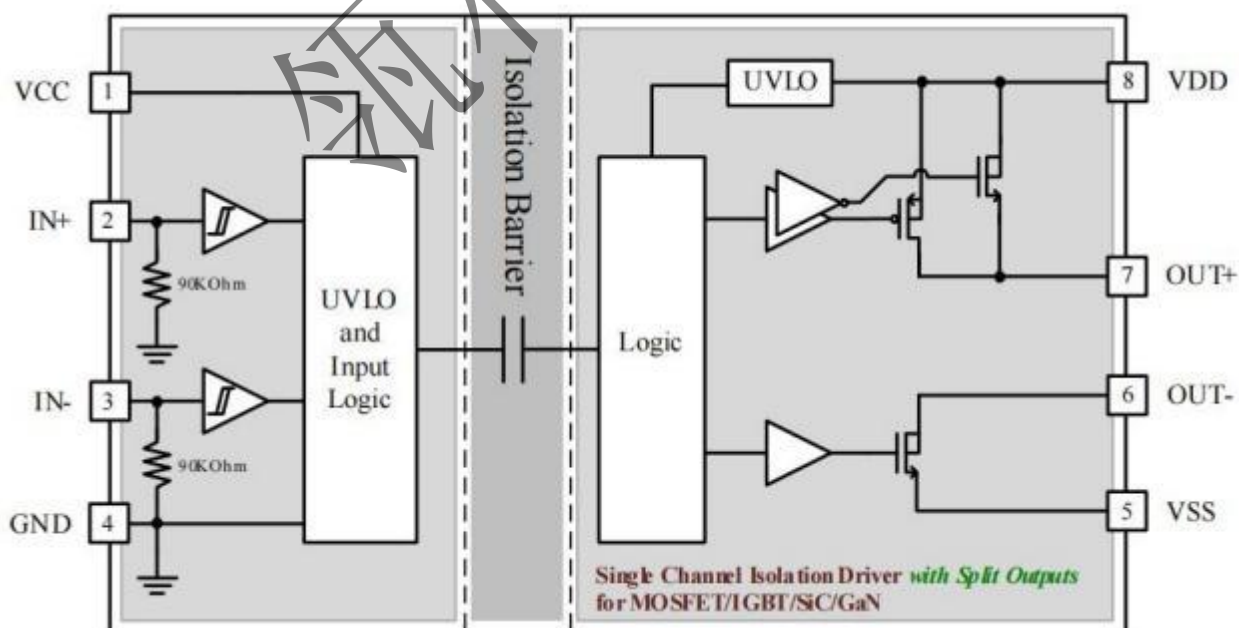
图 27 功能框图
