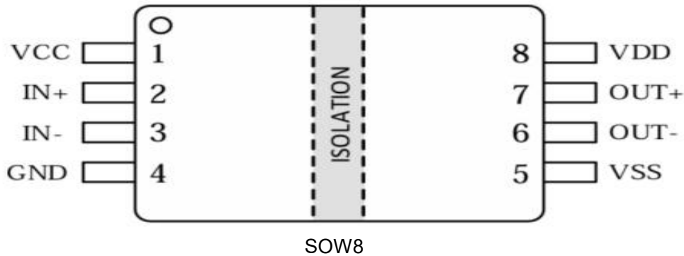
图 2 引脚排列图（顶视图）
