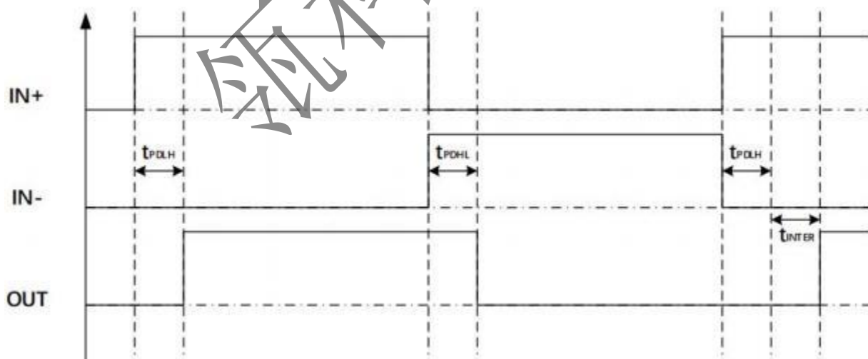
图 23 Interlock 时间的时序图
