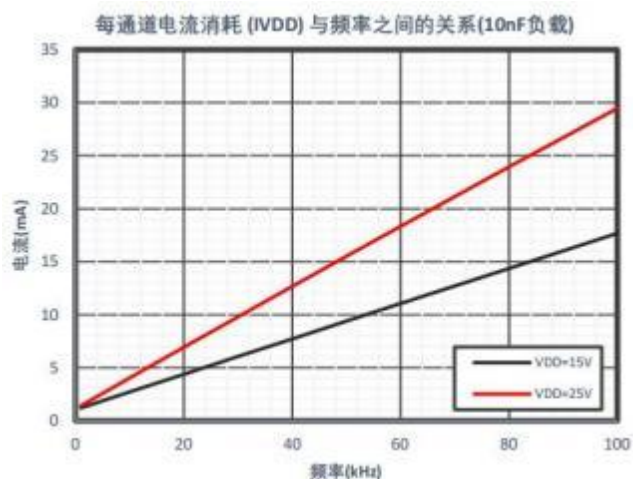
图 5 电流消耗(IVDD)与频率间的关系(10nF 负载)
