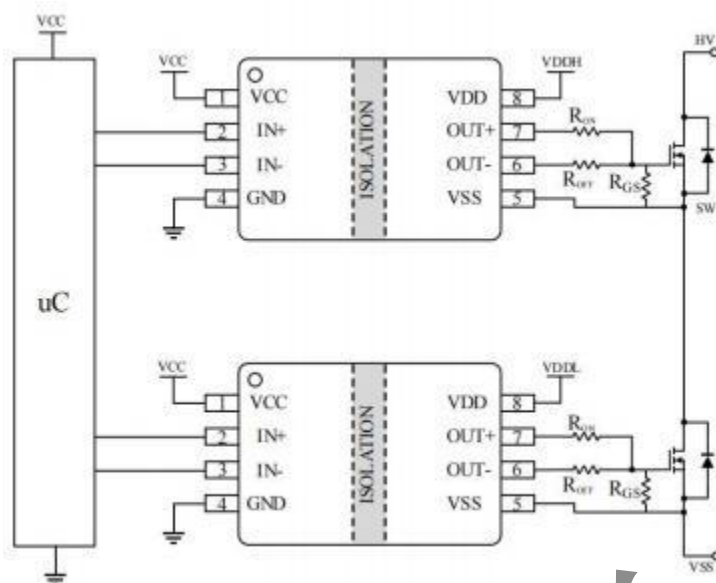
图 1 典型应用图
