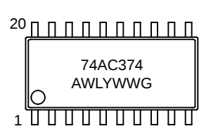
SOEIAJ–20
