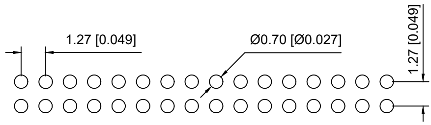
P.C.B LAYOUT
