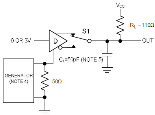
图 5 使能和关断时间 ( t_{PZH} , t_{PSH} , t_{PHZ} )
