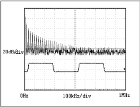
图11：传输20kHz信号时 SP3485EEN+TD驱动器输出波形和FFT图
