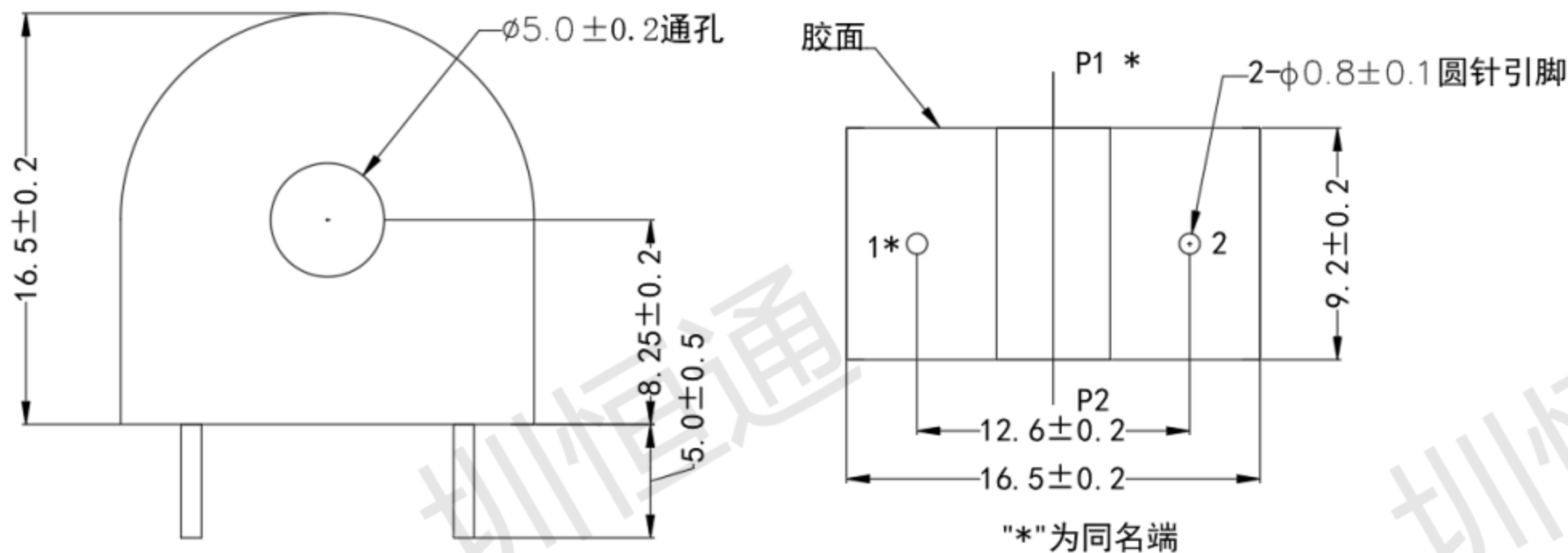
主视图
