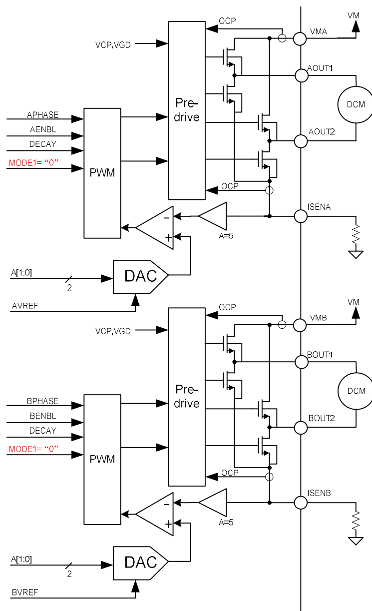
图 4. 马达控制电路
