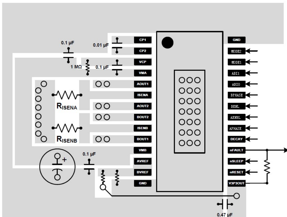
图 9. SS6951A 布局实例
