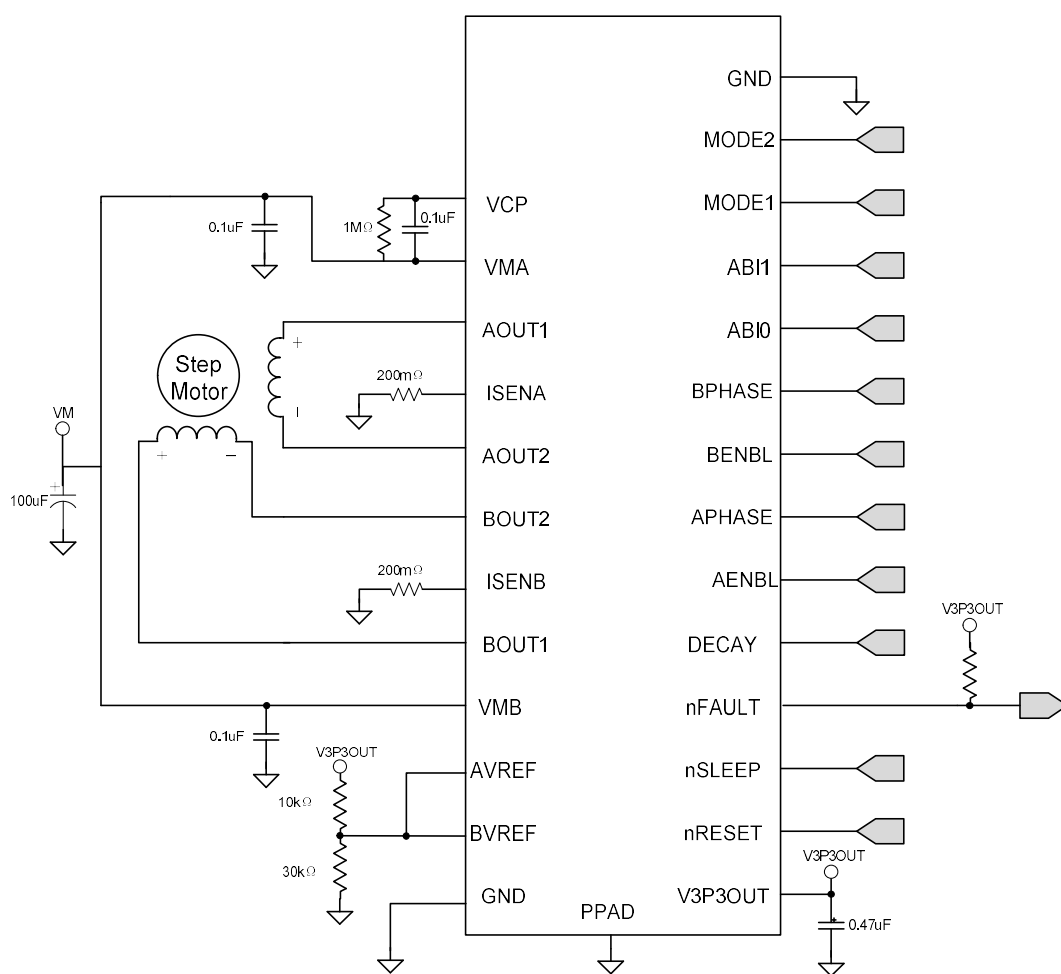
图 6. 典型应用电路一
