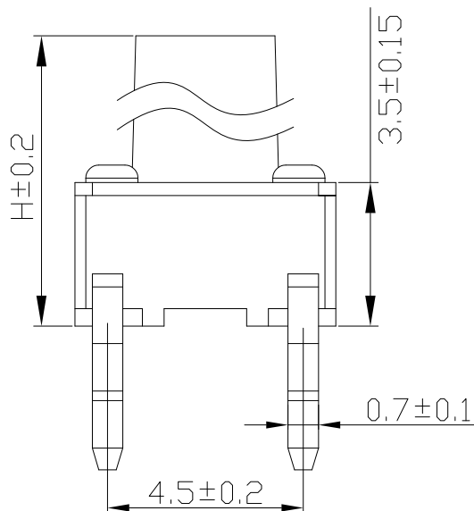
PCB参考图
