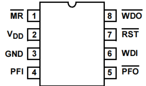
ISL88813 (8 LD SOIC)
