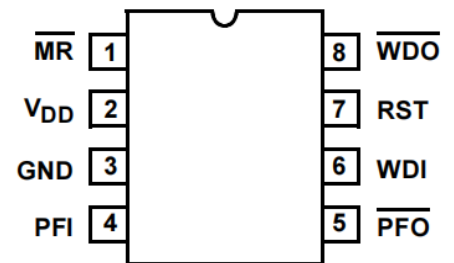
ISL88708 (8 LD SOIC)
