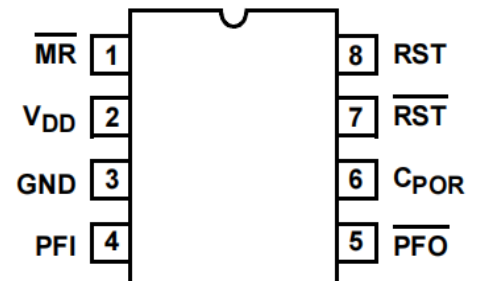
ISL88708 (8 LD SOIC)
