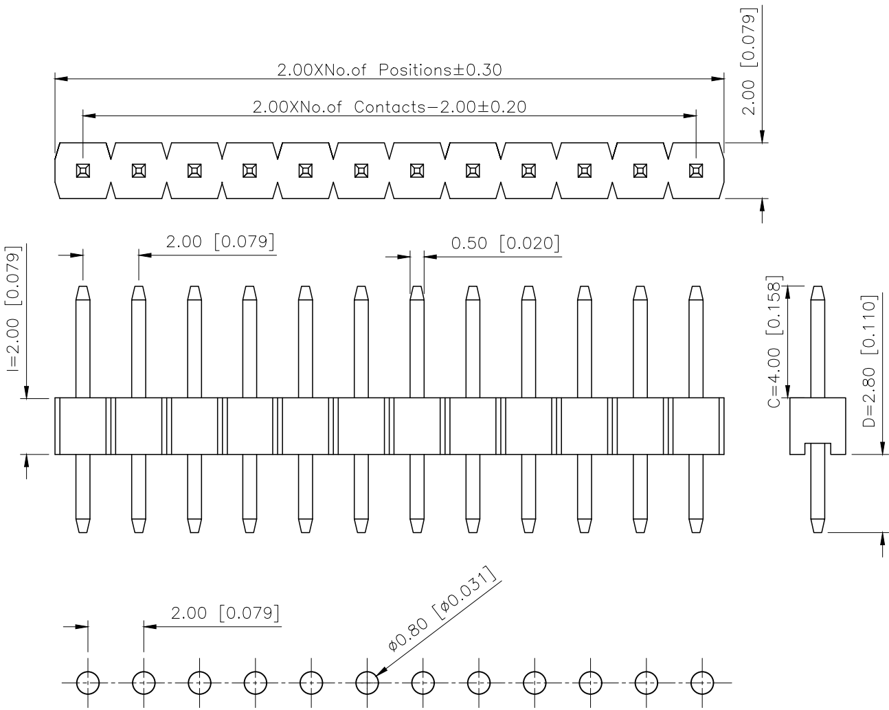
P.C.B LAYOUT
