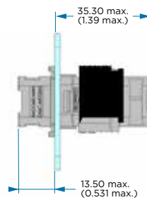
Extender Receptacle
