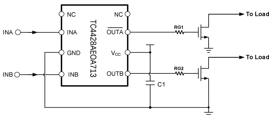
TC4428AEOA713 典型应用电路图
