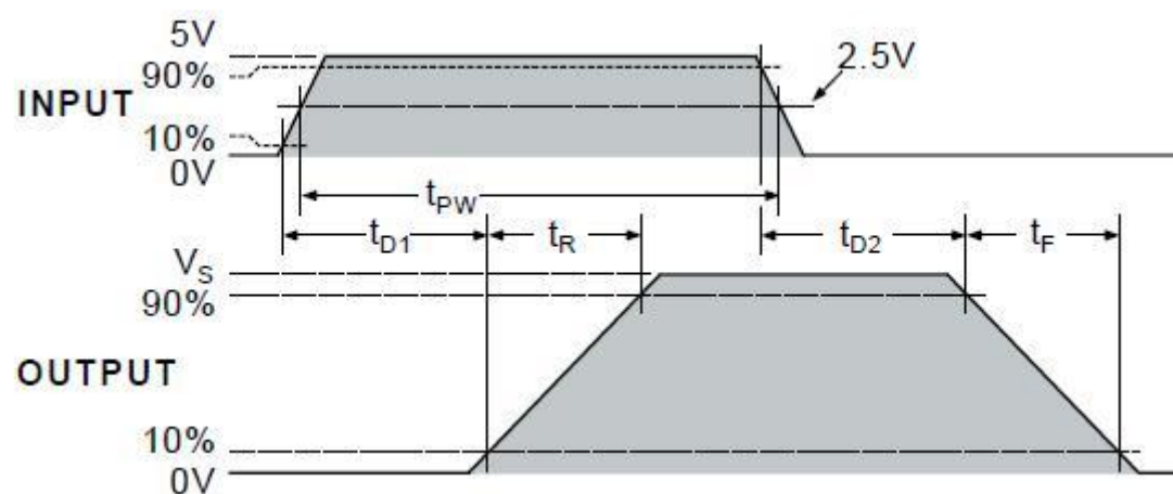
输入输出(B 通道同相)波形图
