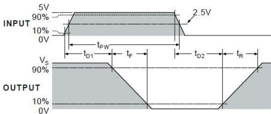
输入输出(A 通道反相)波形图
