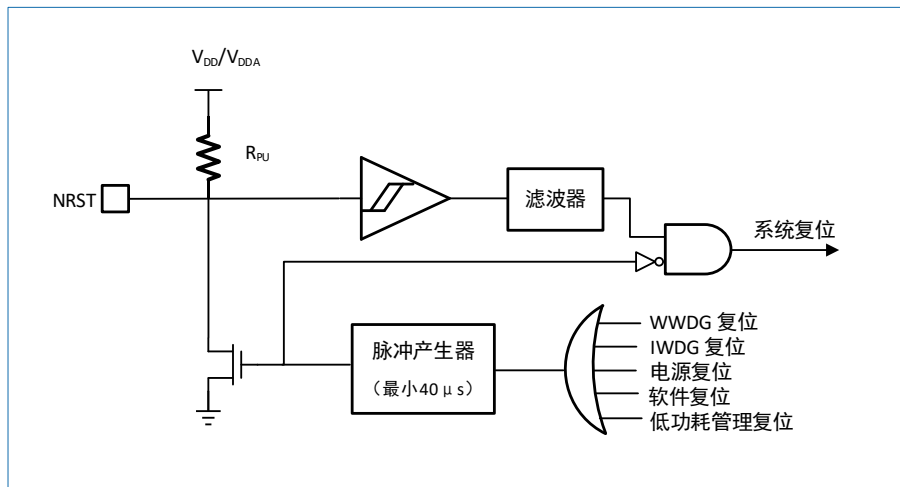
图 3-3 复位电路
