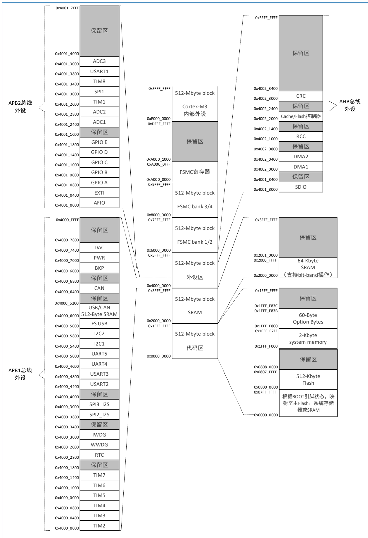
图 3-2 HK32F103xCxDxE 存储器映射表
