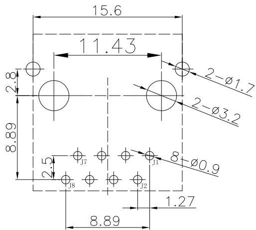
P. C. B参考图
