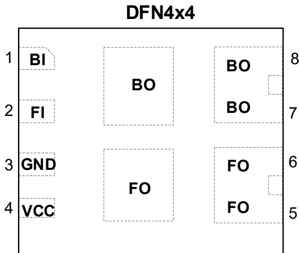
图 1. 顶视图
