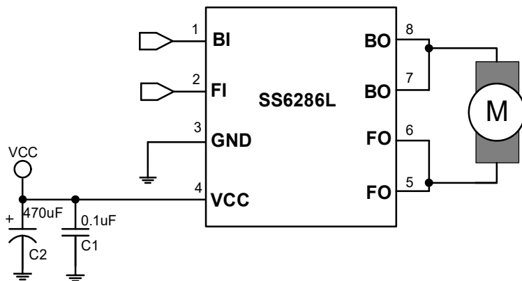
图 4. 应用原理图
