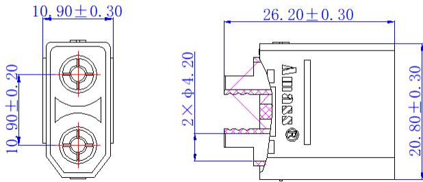
产品尺寸
