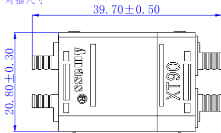
对插尺寸
