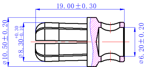
产品尺寸
