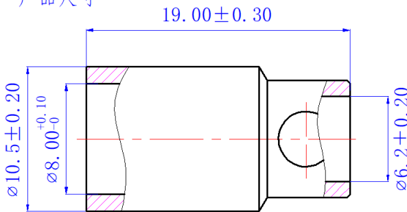
产品尺寸
