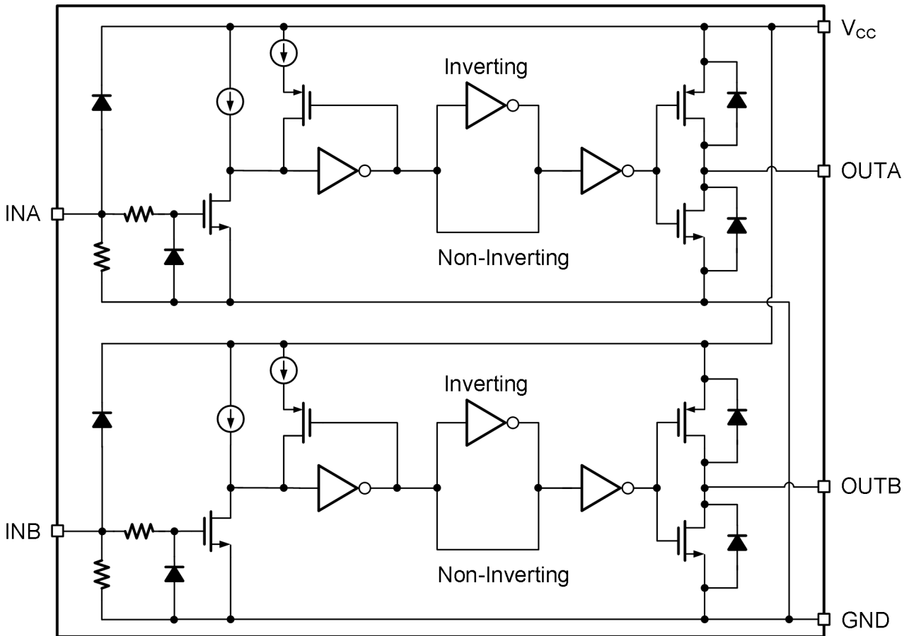
TC4427AEOA713 功能框图
