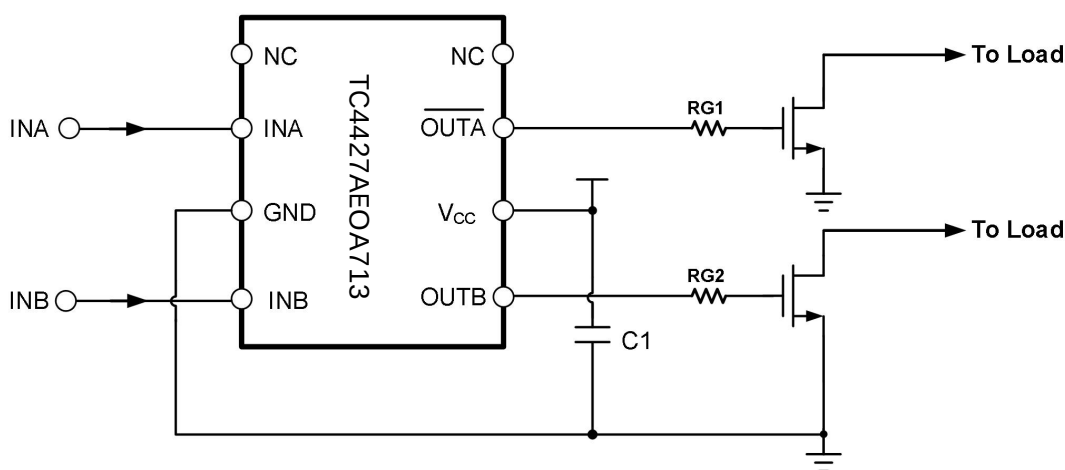
TC4427AEOA713典型应用电路图
