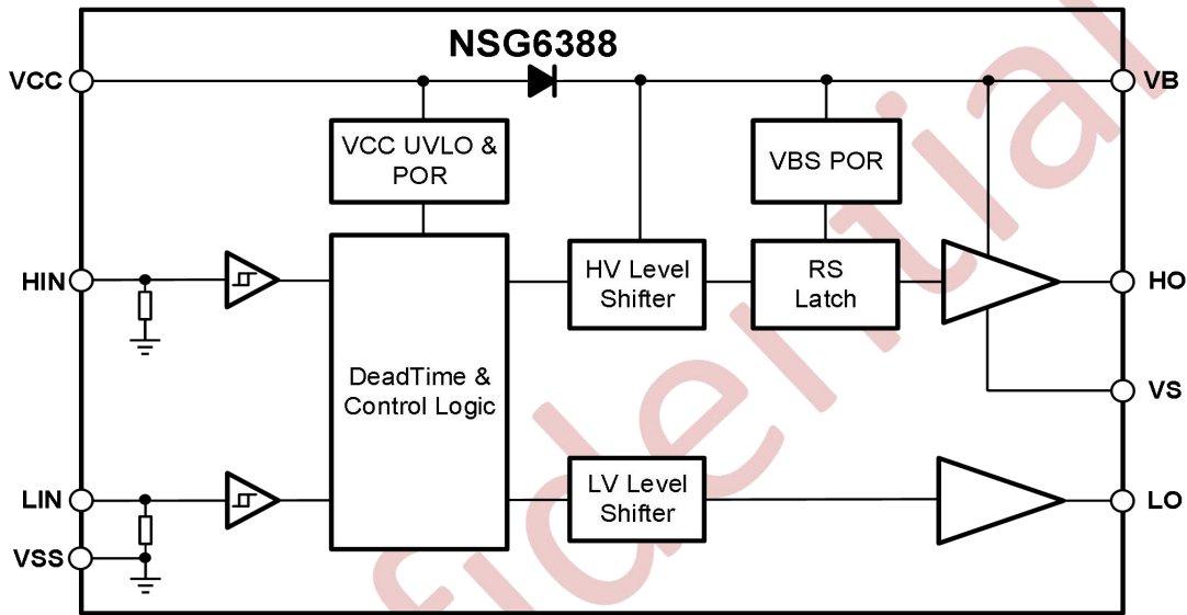
图 10-1 NSG6388 的功能框图
