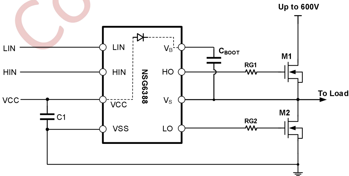
图 10-2 NSG6388 典型应用电路图
