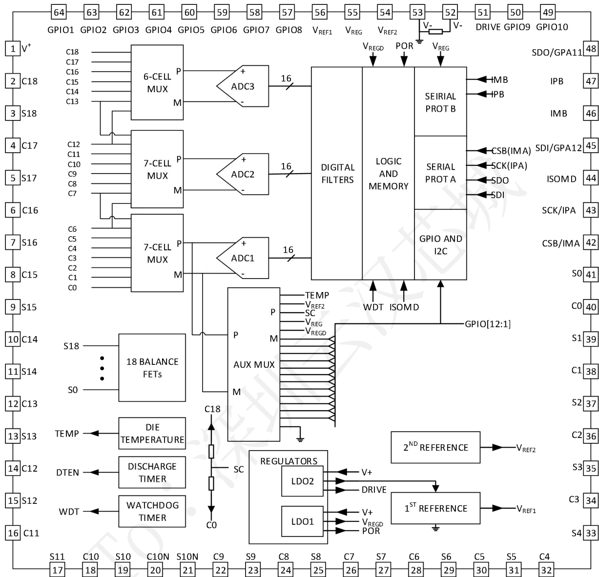
图 5-1：结构框图
