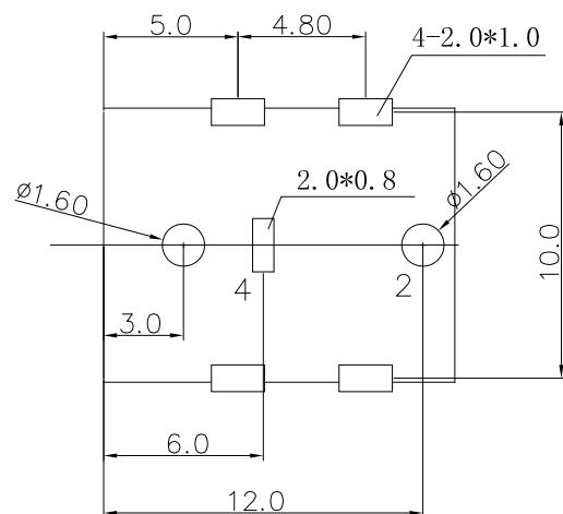
PCB参考图
