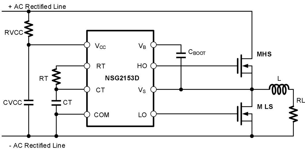
图 10-2 NSG2153D 典型应用电路图
