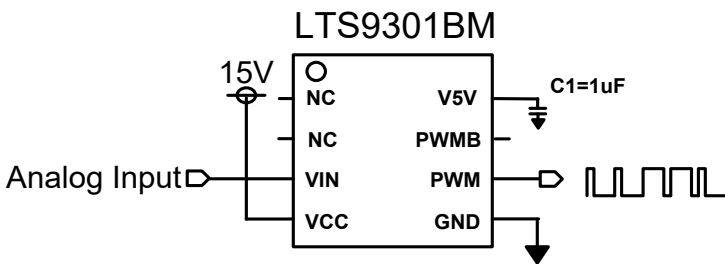
LTS9301B 电压转PWM关系
