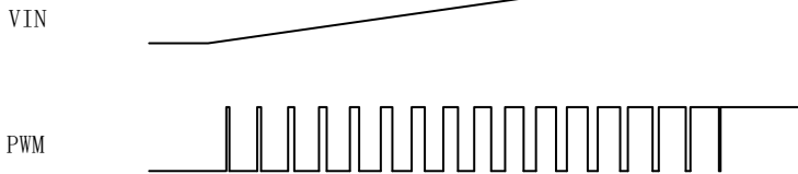
LTS9301BM与LTS9301B输出信号关系
