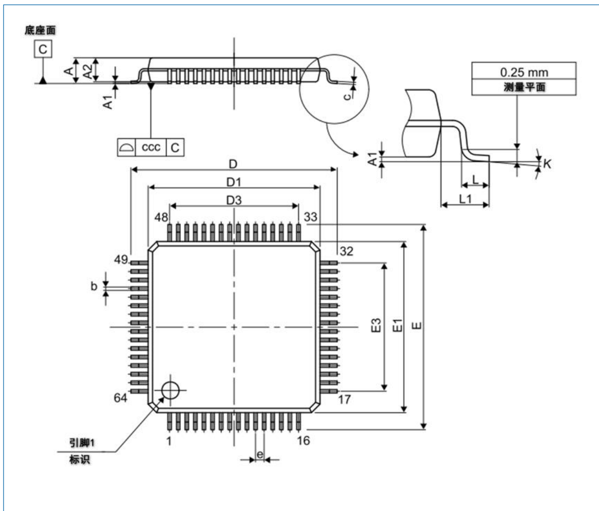
图 7-1 LQFP64 封装尺寸图
