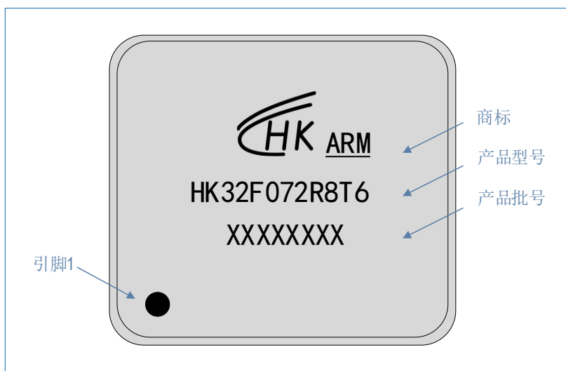
图 7-5 LQFP64 HK32F072R8T6 丝印示例
