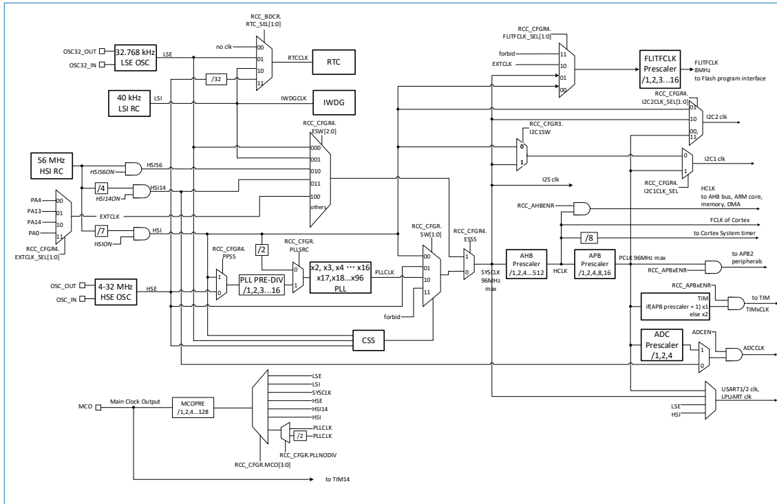
图 3-4 HK32F072x8xB 时钟树
