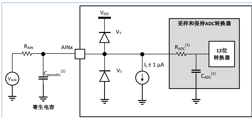
图 4-4 ADC 的典型连接图
