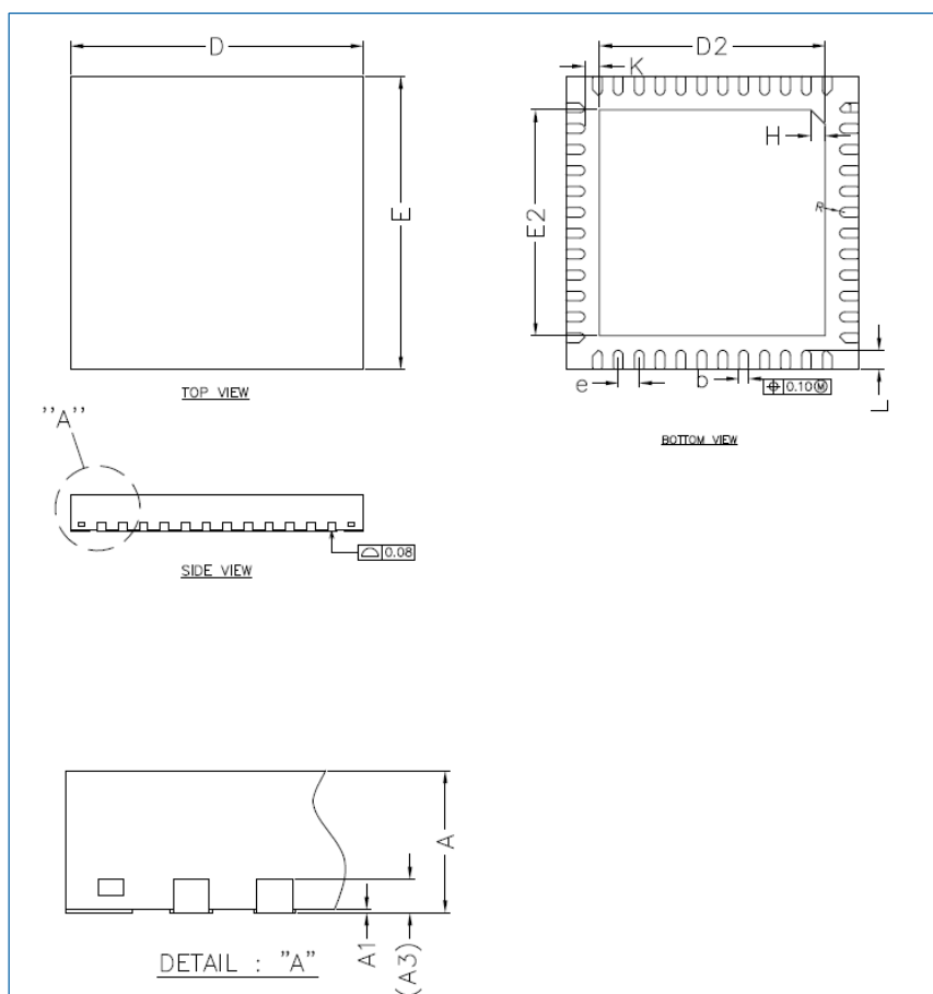
图 7-3 QFN48 封装尺寸图
