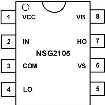
图 7-1 8-脚 SOP8 顶视图
