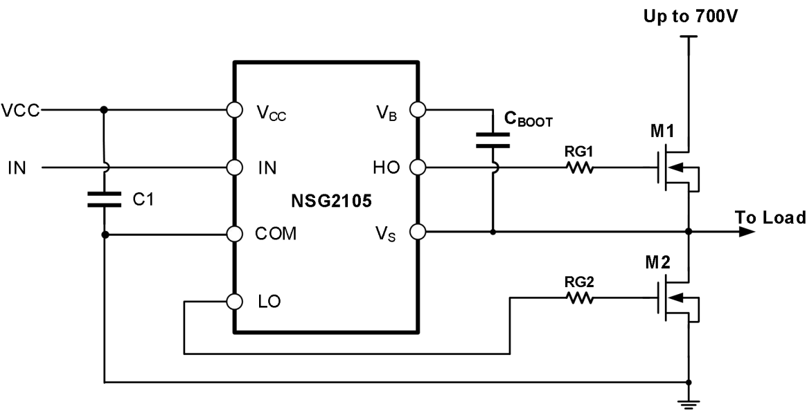
图 10-2 NSG2105 典型应用电路图
