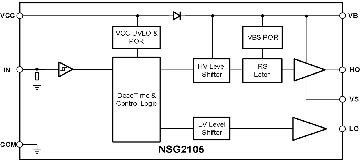
图 10-1 NSG2105 的功能框图
