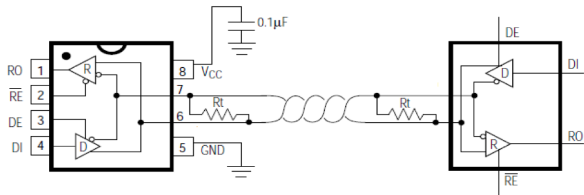
图 1：ST3485EBDR-TD典型半双工应用电路
