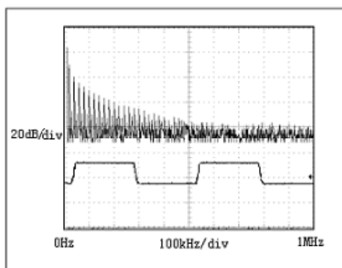
图11：传输20kHz信号时 ST3485EBDR-TD驱动器输出波形和FFT图
