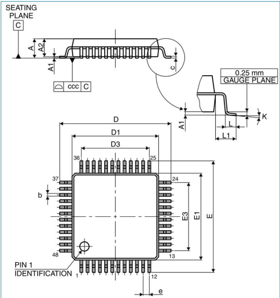
图 6-2 LQFP48 封装尺寸
