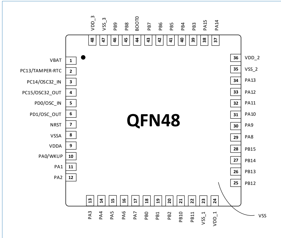
图 5-1 QFN48 封装
