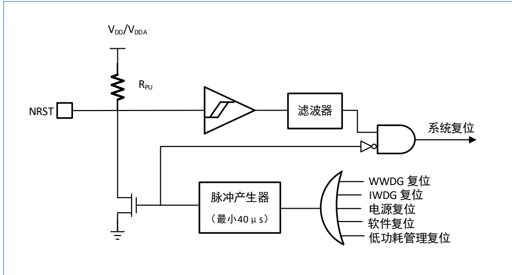
图 3-3 芯片复位
