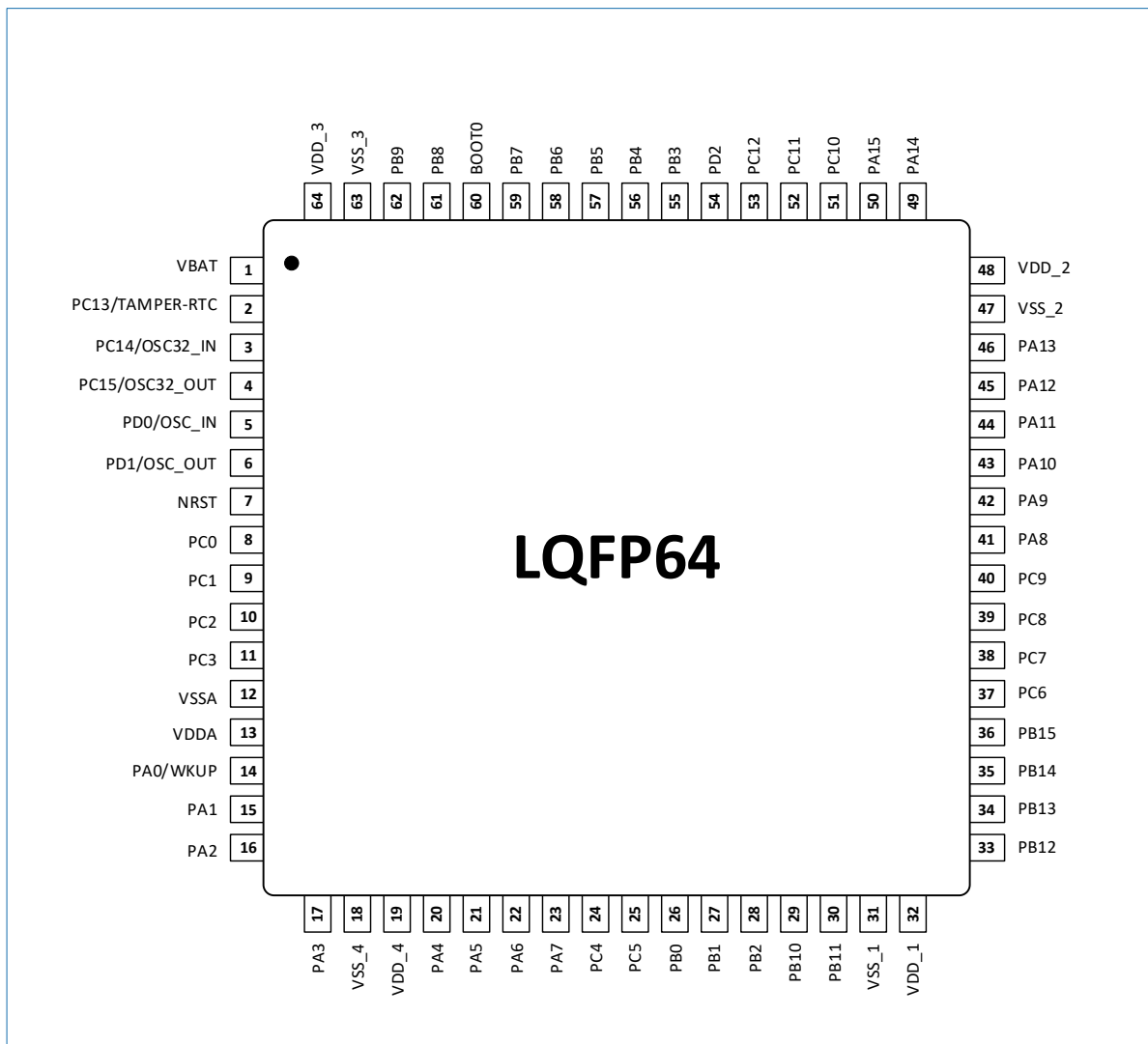
图 5-3 LQFP64 封装
