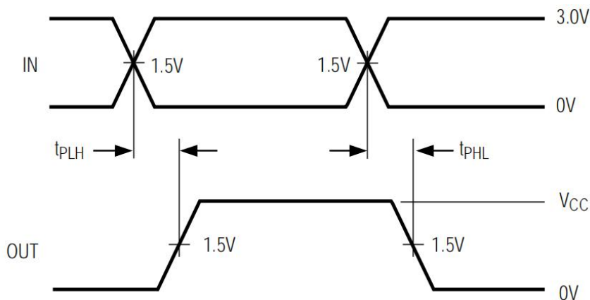
图3 接收器传输延迟时序图
