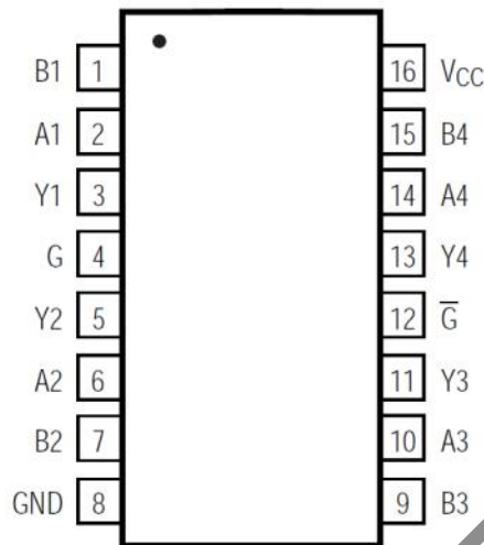
图 2 引脚排列图（顶视图）
