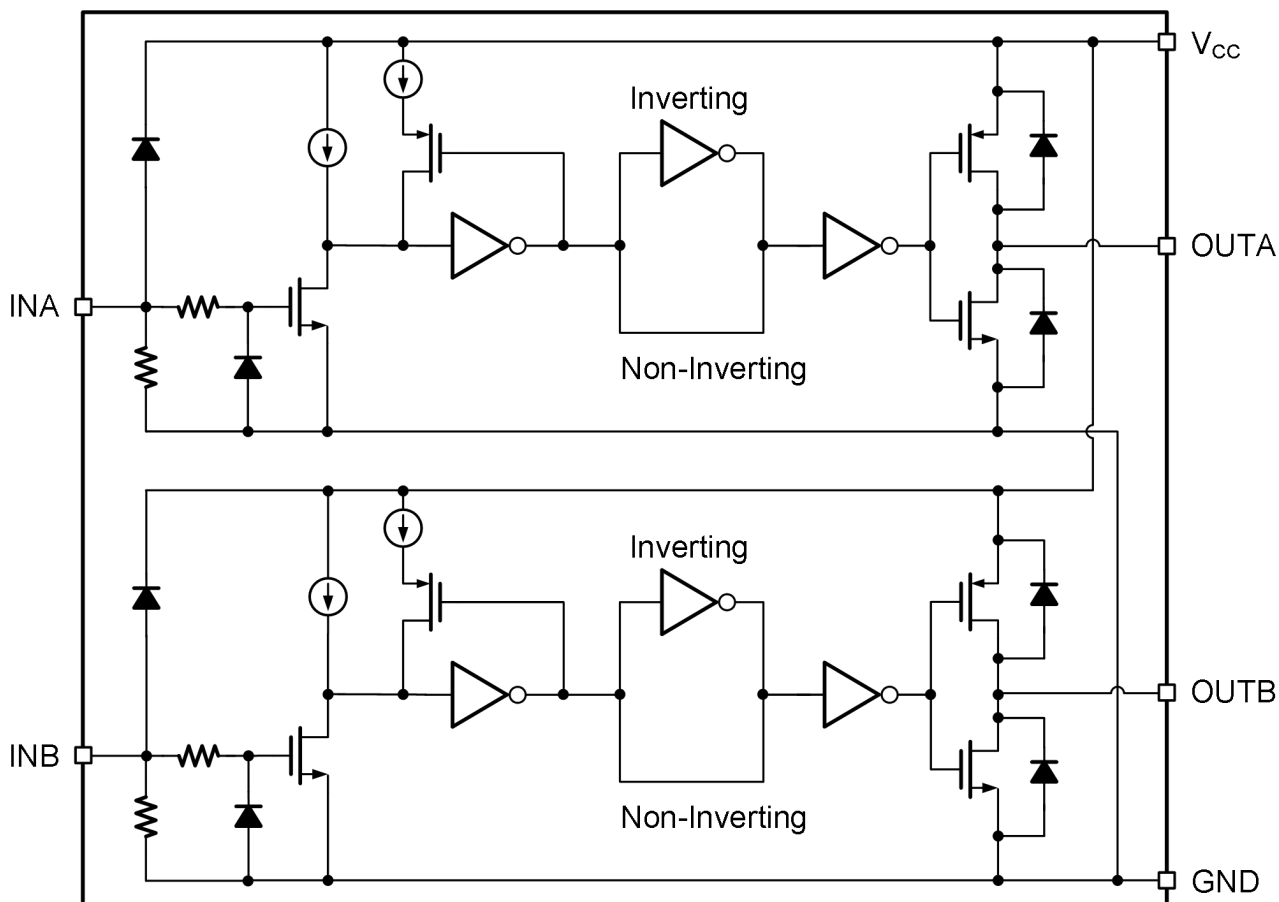
IR4427STRPBF功能框图
