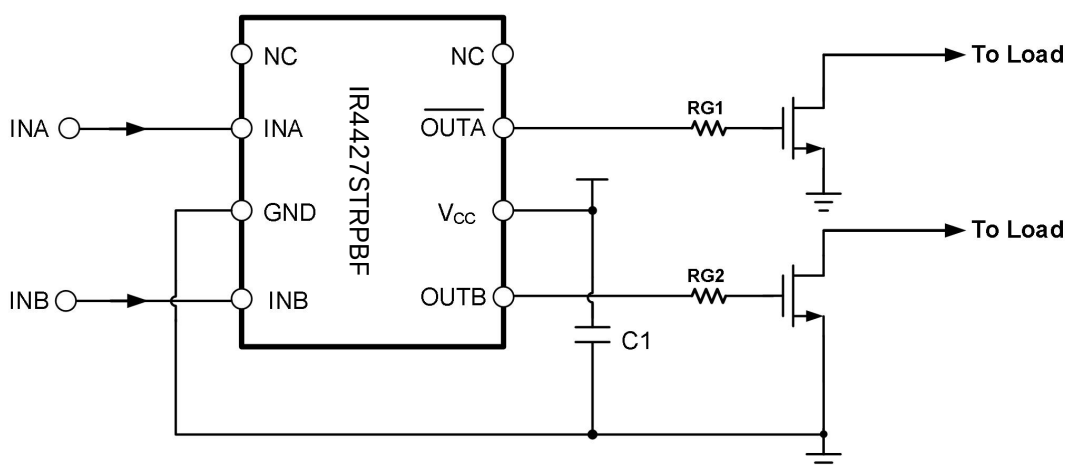
IR4427STRPBF 典型应用电路图
